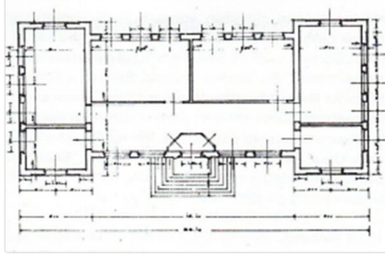
Grsel 1- Edirne Karaağaç İbtidai Mektebi Planı (Yıldırım Yavuz)
