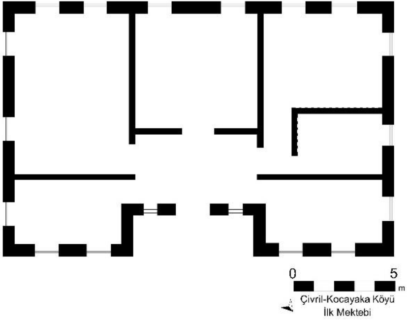
Görsel 34- Kocayaka İlk Mektebi Plânı (Kadir Türkmen)
