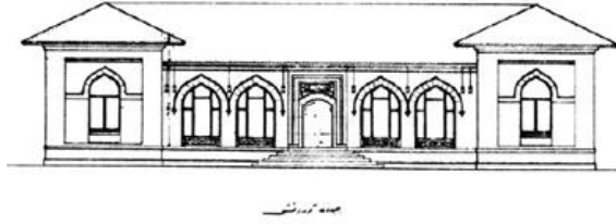
2. Edirne Karaağaç Mektebi, cephe
