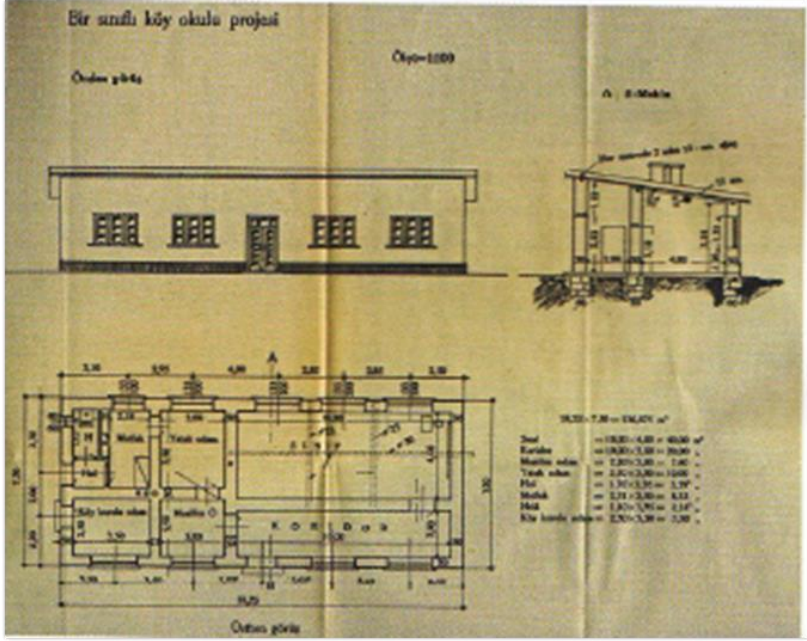
Görsel 6- Köy Eęitmenleri Kanununa İstinaden Hazırlanan Tip Proje (Nurřen Kul)
