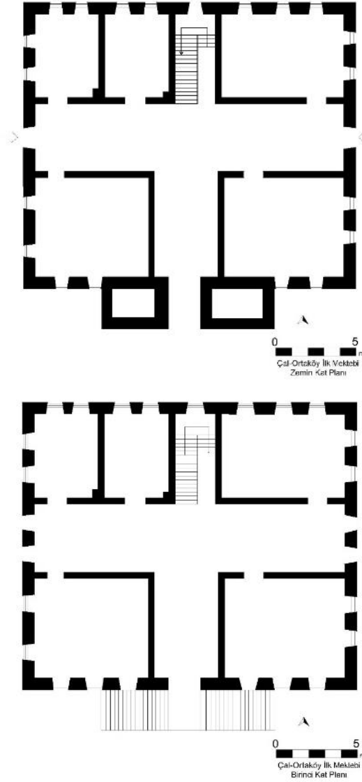
Görsel 10-11- Ortaköy İlk Mektebi Zemin ve Birinci Kat Plânı
