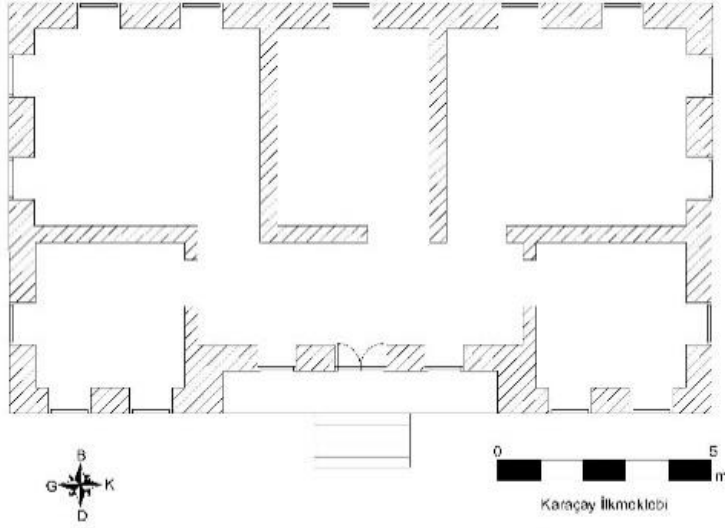
Görsel 29- Karaçay İlk Mektebi Plânı (Kadir Türkmen)
