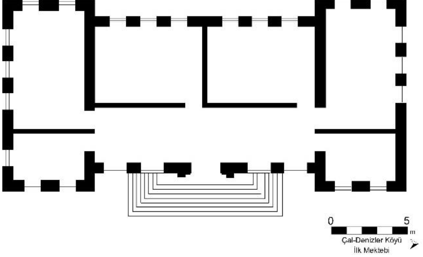
Görsel 24- Denizler İlk Mektebi Plânı (Kadir Türkmen)
