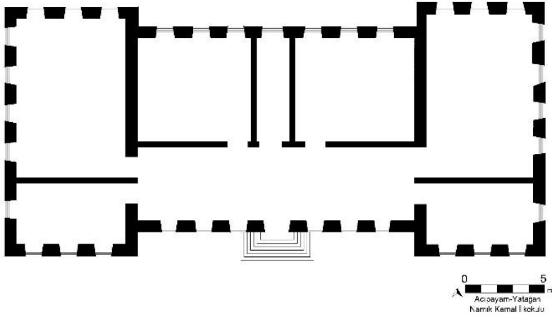
Görsel 19- Yatağan Namık Kemal İlk Mektebi Plânı (Kadir Türkmen)
