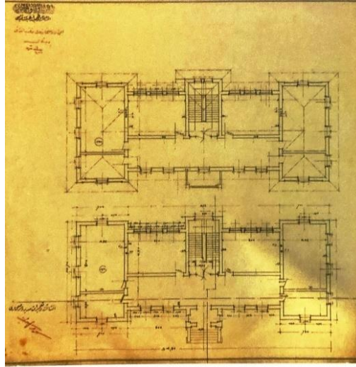
Görsel 37- Mimar Kemalettin’e Ait Altı Derslikli Okul Projesi 40
