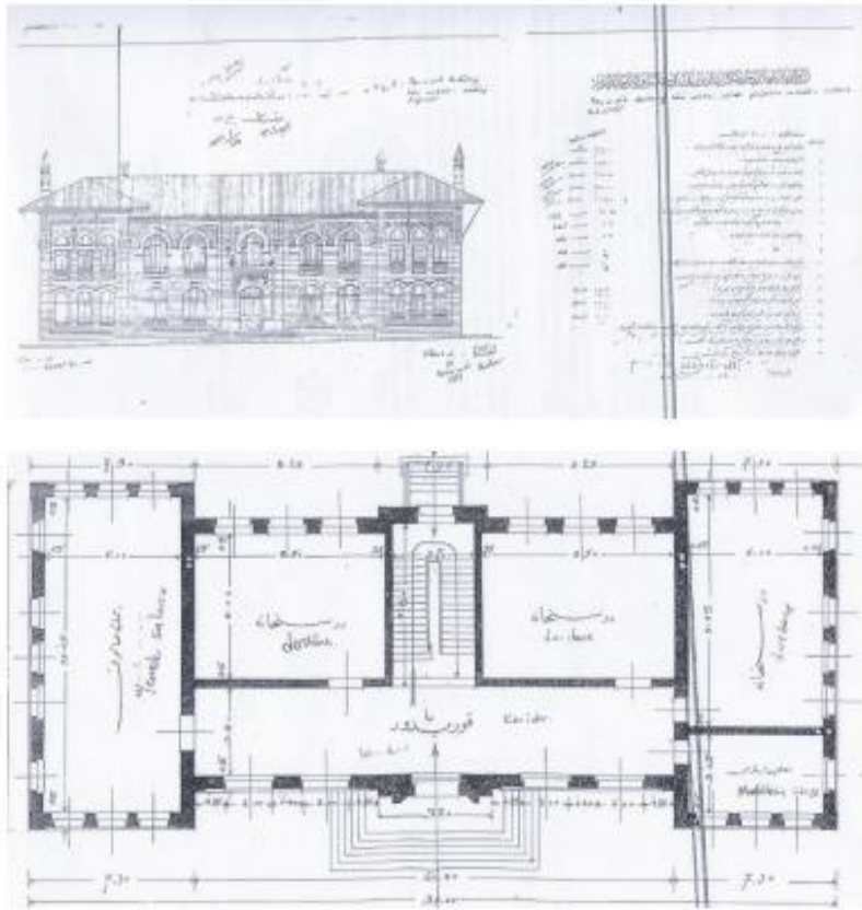
Görsel 4-5- Mukbil Kemal Bey'in 'Beş ve Altı Dershaneyi Hâvi Mekteb-i İbtidai Projesinin Mikdar-ı İmâlat Cetvelidir.' başlıklı projesi (Alper Atıcı)
